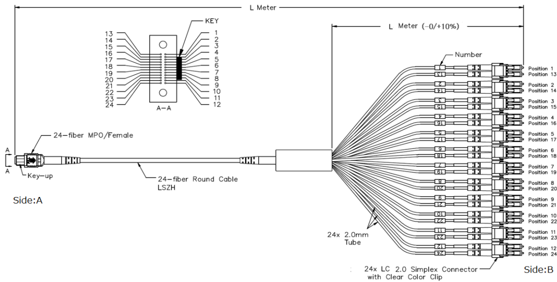
付図3. 例) ALP-24FOM4-MPOF/12DLC-END-△M
