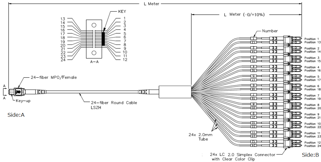
付図3. 例) ALP-24FOM3-MPOF/12DLC-END-△M
