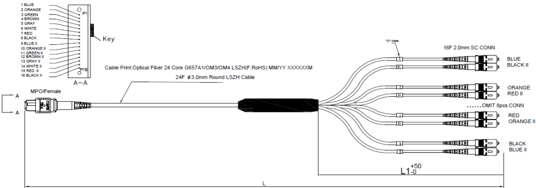
付図4. 例) ALP-24FOM3-16MPOAM/16SC-END-△M
