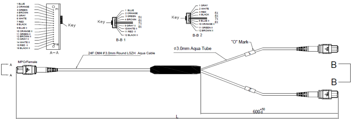
付図3. 例) ALP-24FOM3-16MPOAF/2x12MPOF-BR2-△M
